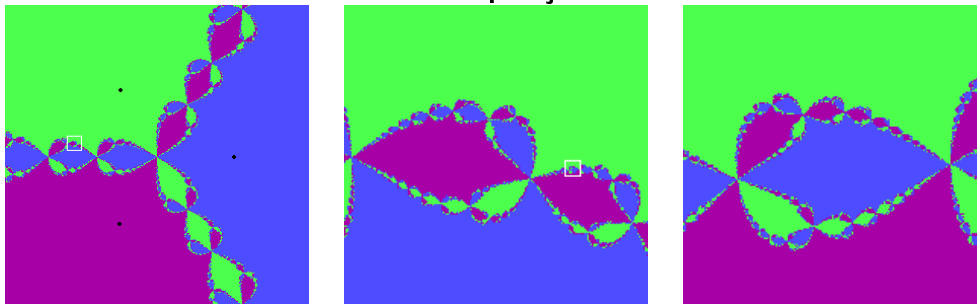
Fractaalplaatje 2:
